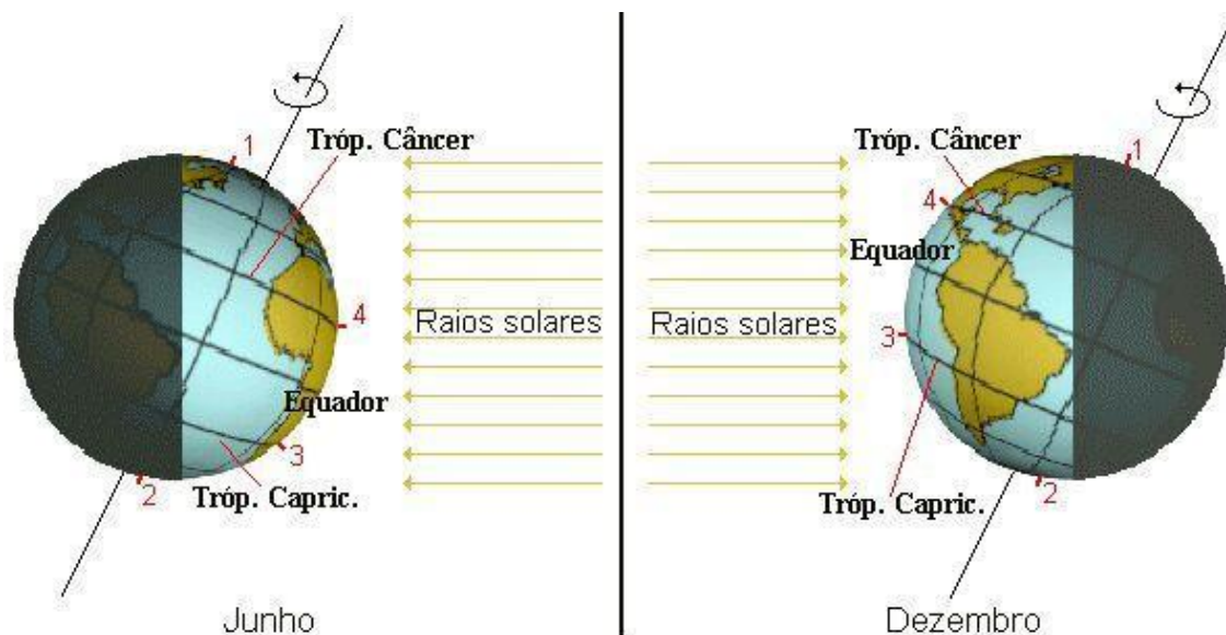
Figura 2 - Representação da Incidência Solar em relação ao ângulo de inclinação do eixo de rotação da Terra
