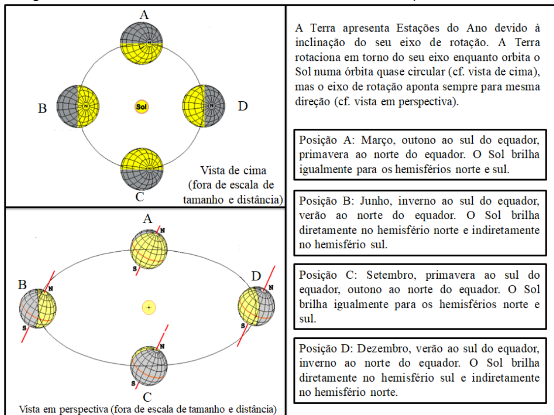
Figura 1 - Posicionamento da Terra em torno do Sol, no período de um ano
