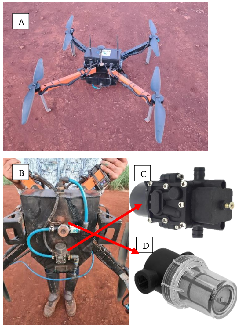
Figura 2.1. A: Visão geral do RPA visto por cima, B: Visão geral do RPA visto por baixo, C: Bomba do tipo peristáltica, D: Filtro de bomba de malha de 100 mesh. Foto: Silva, A.S. (2022).
