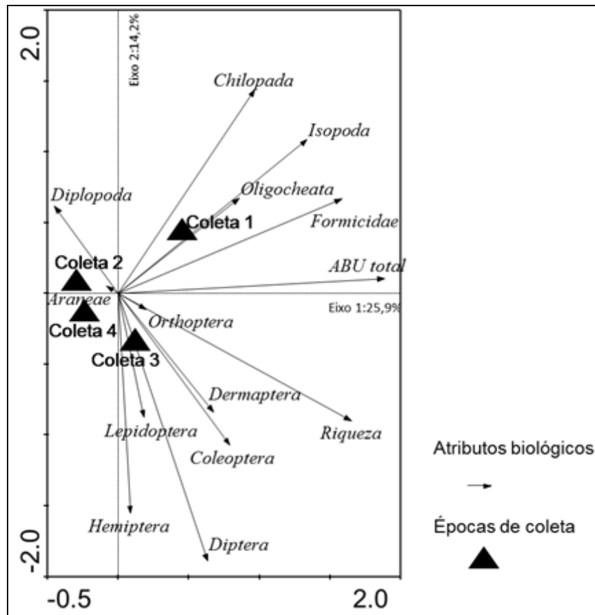
Figura 10 - Análise de Componentes Principais dos grupos das macrofauna encontrados, abundância total e riqueza em relação às épocas de coleta
