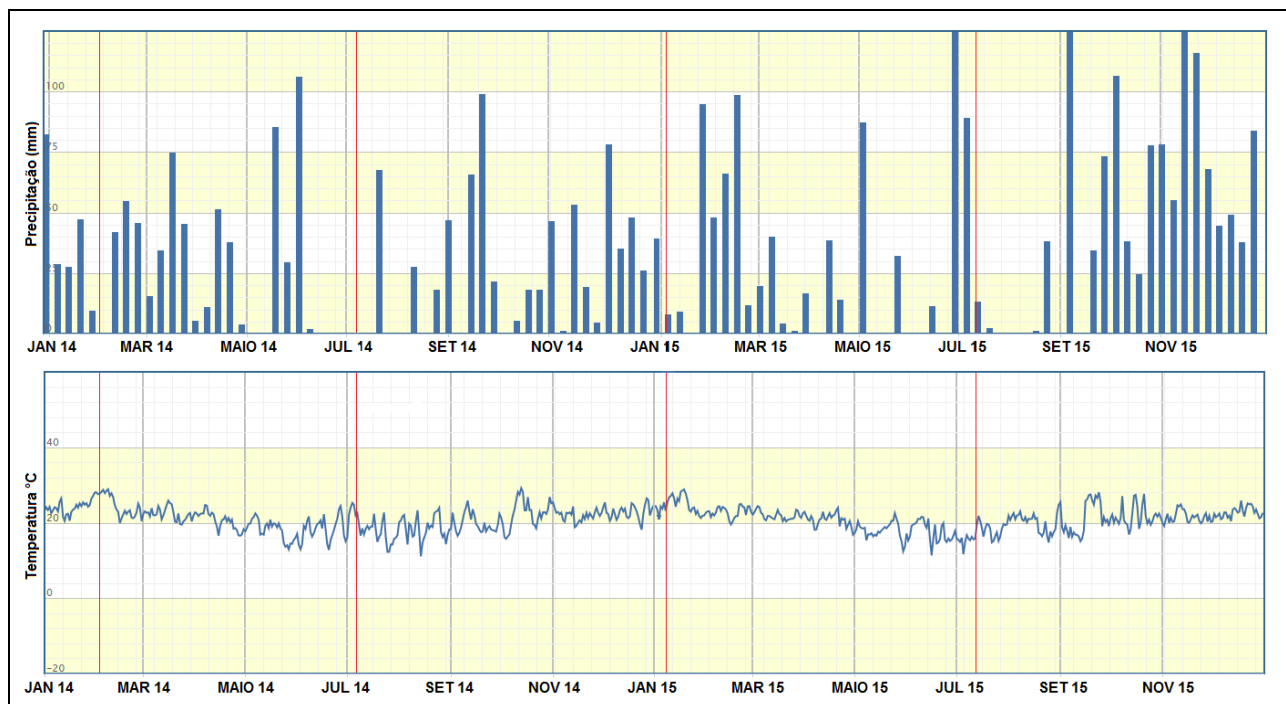
Figura 2 - Precipitação e temperatura do ano de 2014 e 2015 (dados da Estação Automática de Ibaiti/PR – INMET), demarcado em vermelho as datas das coletas.
