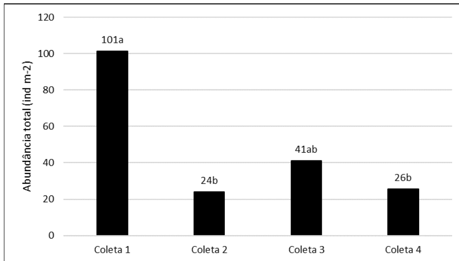
Figura 8 - Dados de abundância total nas diferentes épocas de coleta transformados em \log(x+1) e submetidos aos teste de médias Fisher LSD ( p < 0,05 ).
