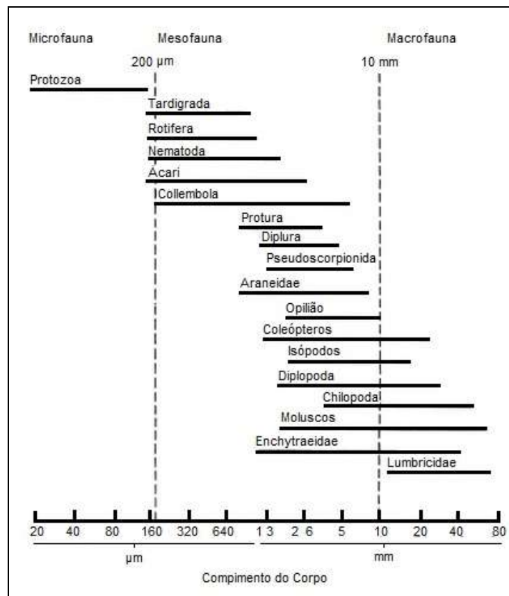
Figura 1- Classificação por comprimento do corpo da fauna edáfica de climas temperados (adaptado de Wallwork 1970).
