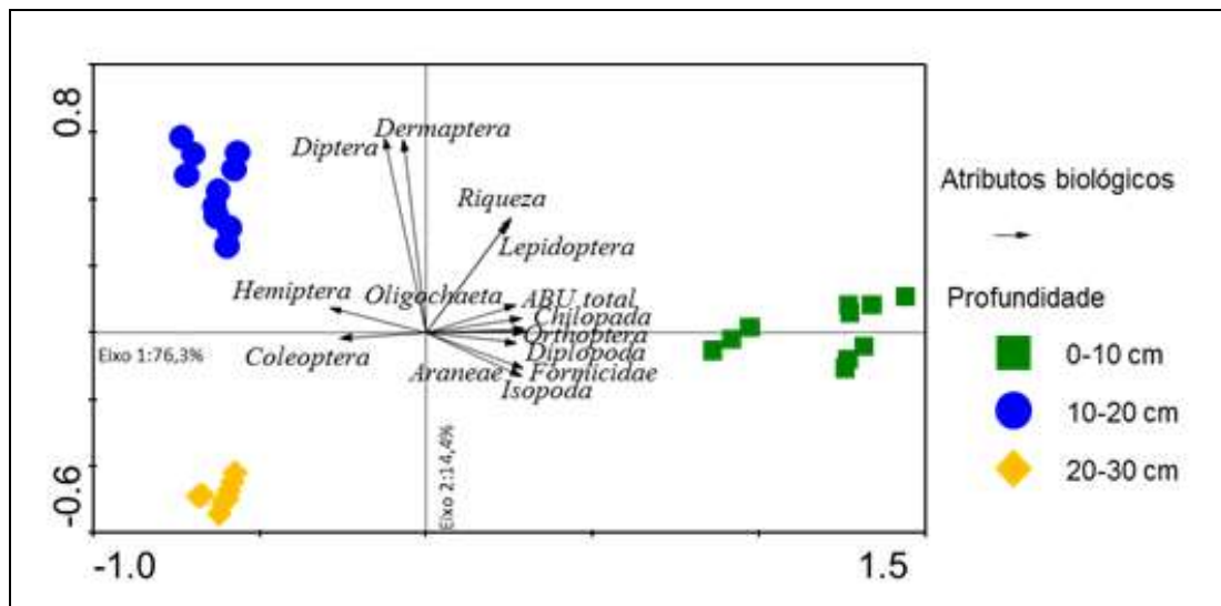
Figura 9 - Análise de Componentes Principais dos grupos das macrofauna encontrados, abundância total e riqueza em relação às diferentes profundidades amostradas.
