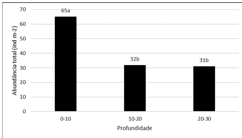
Figura 7 - Dados de abundância total nas diferentes profundidades transformadas em \log(x+1) e submetidas aos testes de médias Fisher LSD ( p < 0,05 ).
