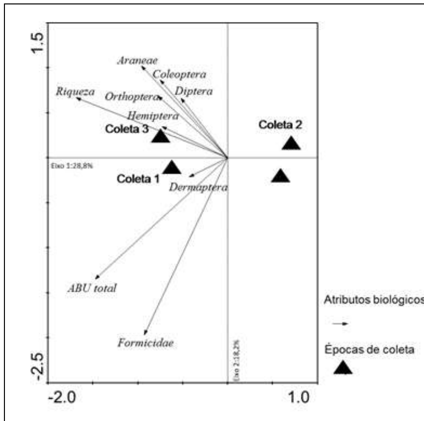
Figura 16 - Análise de Componentes Principais dos grupos das macrofauna encontrados, abundância total e riqueza em relação às épocas de coleta para armadilhas Pitfall em um sistema de cultivo orgânico de cana-de-açúcar, Jaboti PR.
