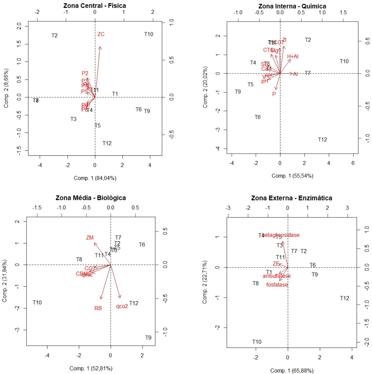
Figura 4. Gráficos de autovetores dos dois primeiros componentes principais agrupados por tipo de variável.
