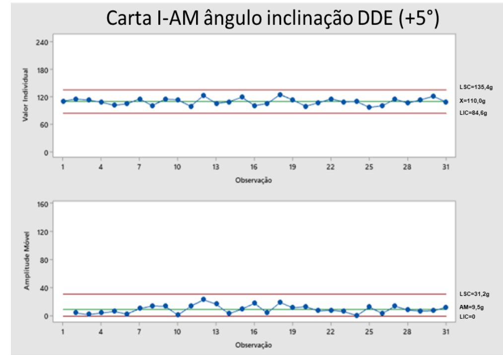
Figura 20. Teste de bancada do Dosador Dupla Esteira em aclave (+5°).
