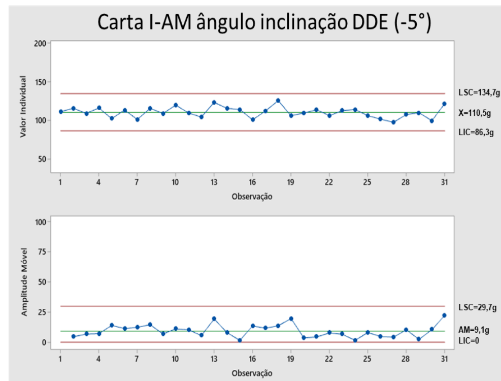
Figura 24. Teste de bancada do Dosador Dupla Esteira em declive de (-5°).
