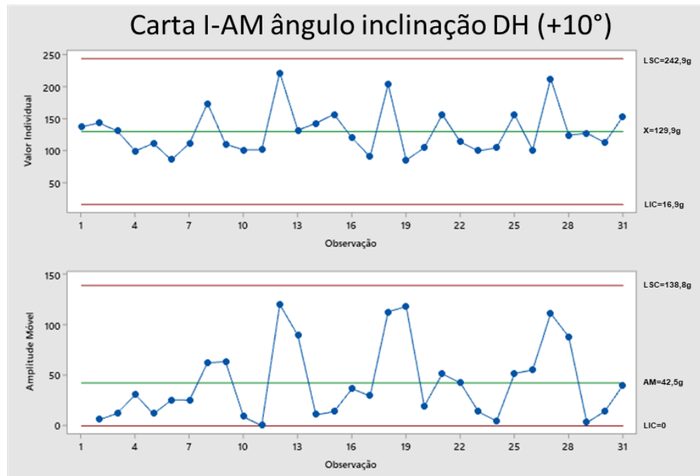
Figura 21. Teste de bancada do Dosador Helicoidal em active (+10°).
