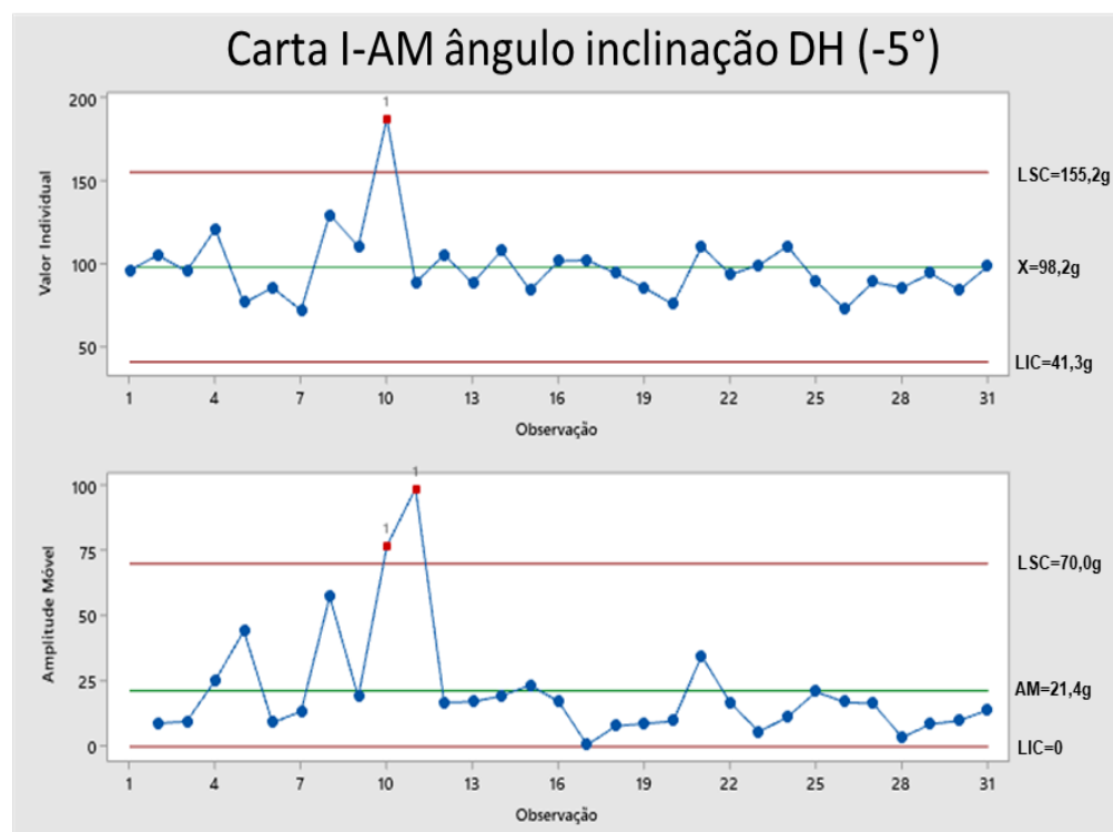
Figura 23. Teste de bancada do Dosador Helicoidal em declive (-5°).
