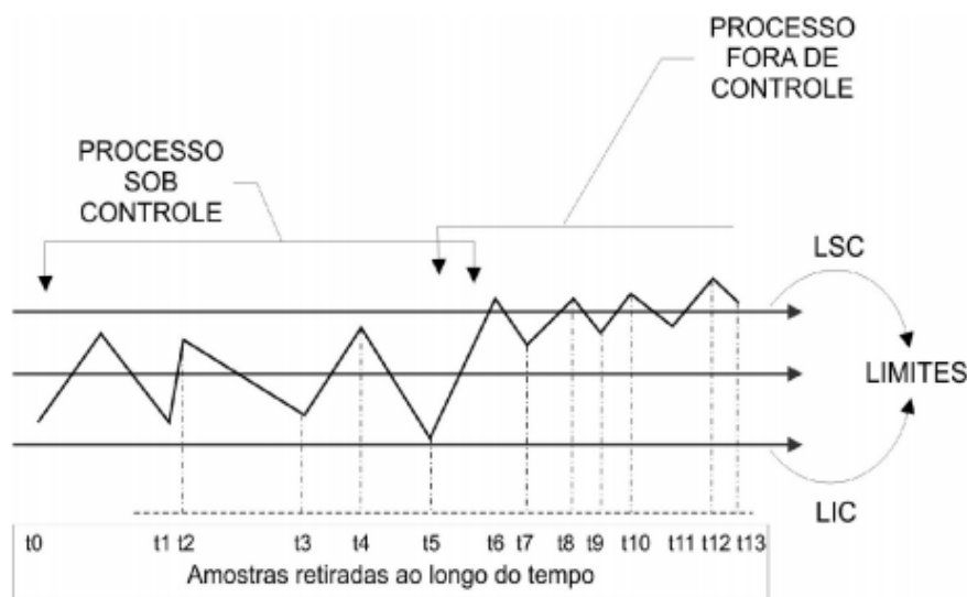
Figura 4. Representação gráfica de processos sob controle e fora de controle.
