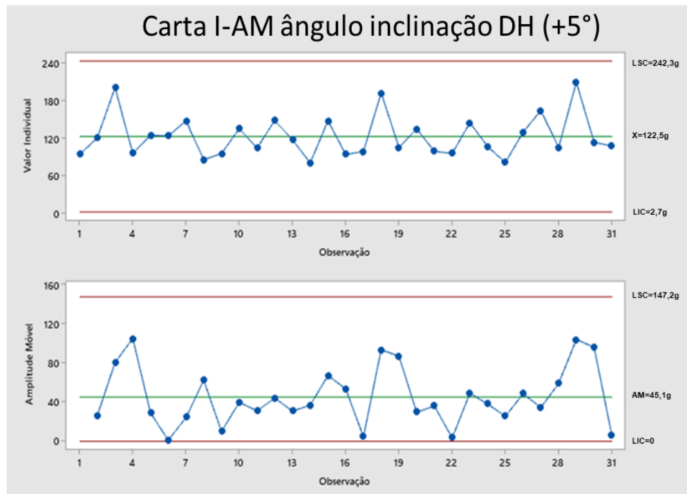
Figura 19. Teste de bancada do Dosador Helicoidal em aclave (+5°).
