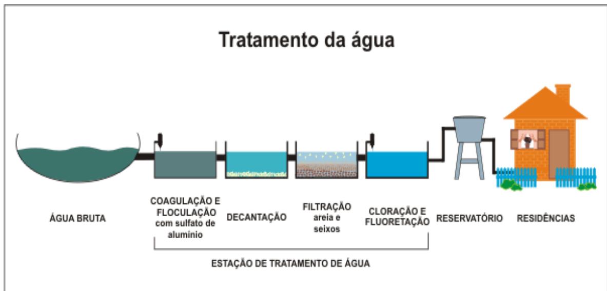
Figura 2: Sistema de Tratamento de Água para Consumo Humano
