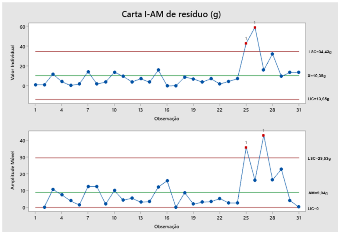
Figura 14. Quantidade de fertilizante passante na peneira p35 ( 0,5 \text{ mm g}^{-1} ).
